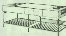
生徒用料理実習台 PT-B4 W210×D90×H80cm 本 ¥245,000 ※コンセント付 ※ガステーブル付
